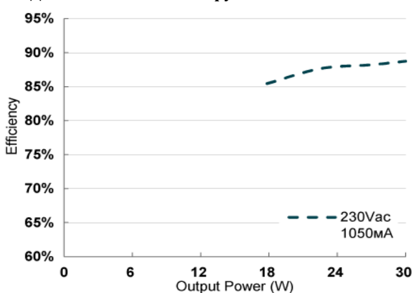
КПД в зависимости от нагрузки
