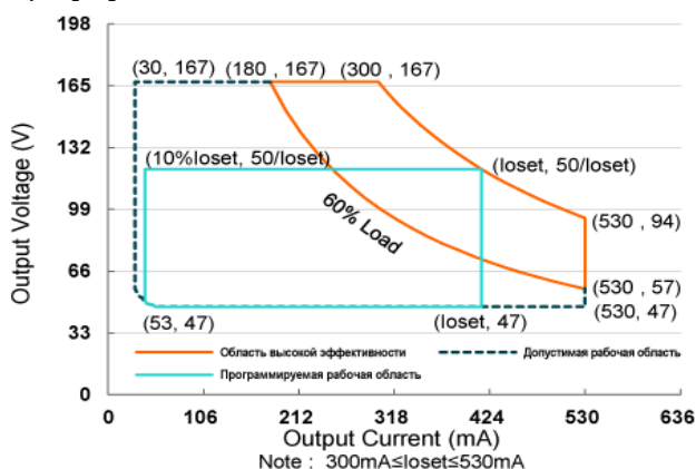
U/I график с областью Постоянная мощность
