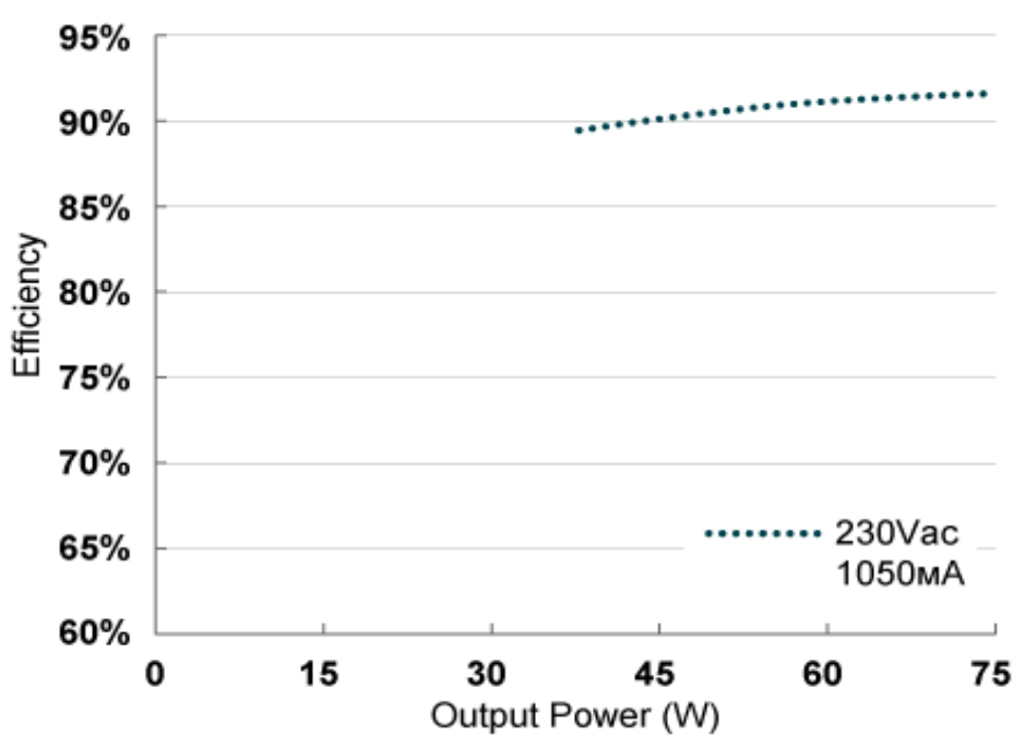
КПД в зависимости от нагрузки
