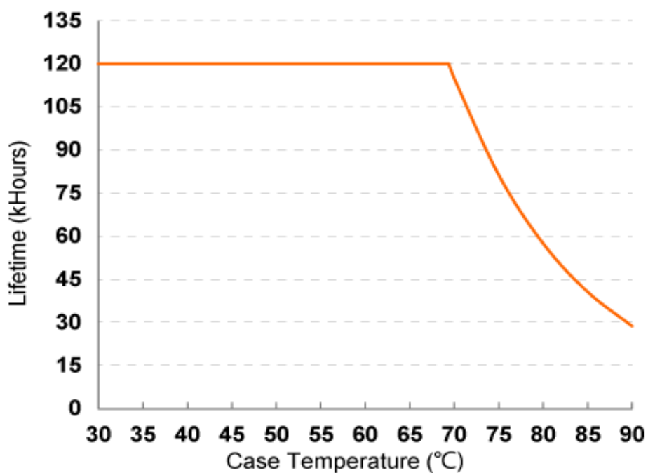
Срок службы / Температура на БП (T c )
