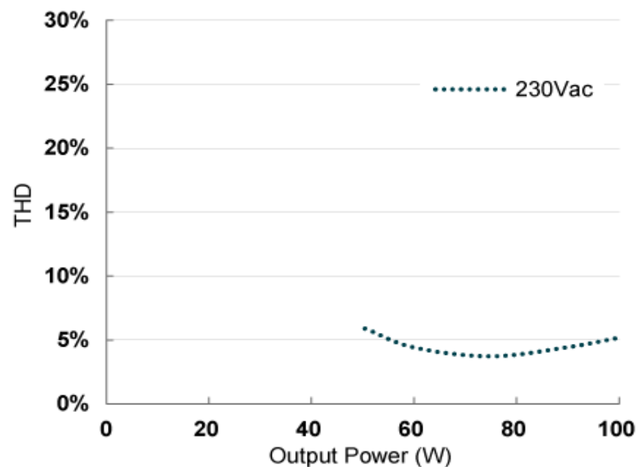
Полные гармонические искажения
