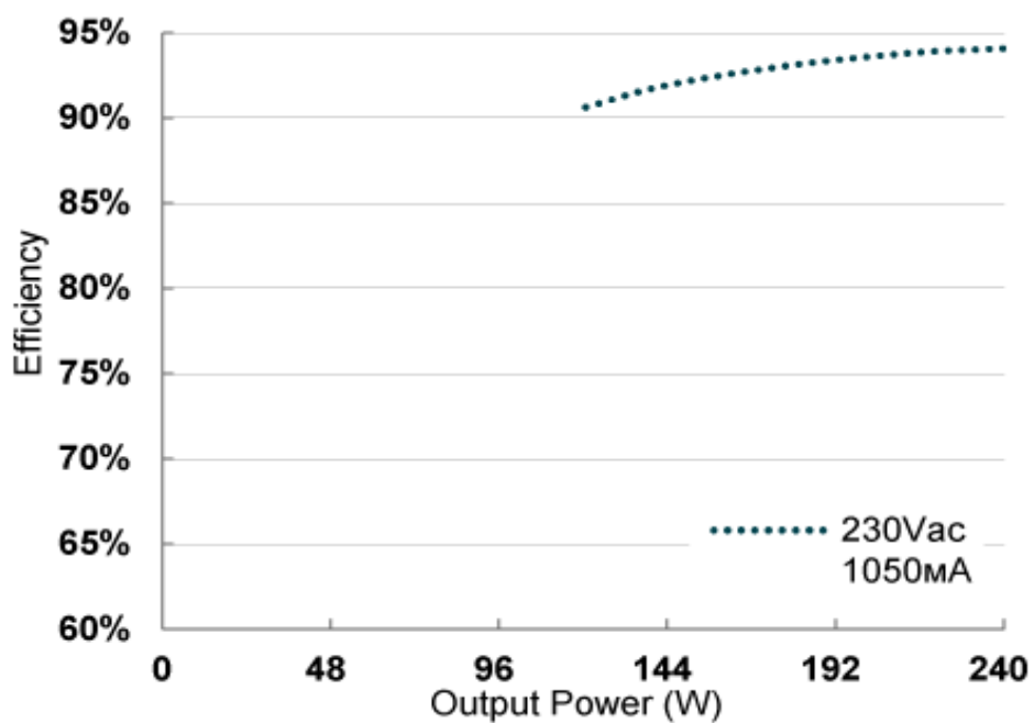
КПД в зависимости от нагрузки
