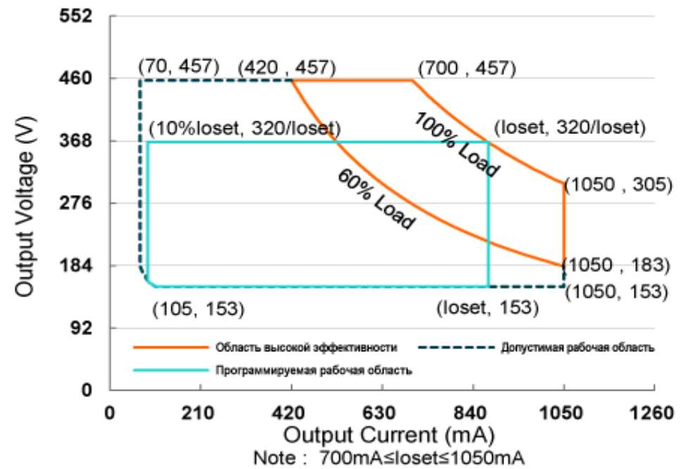
U/I график с областью Постоянная мощность
