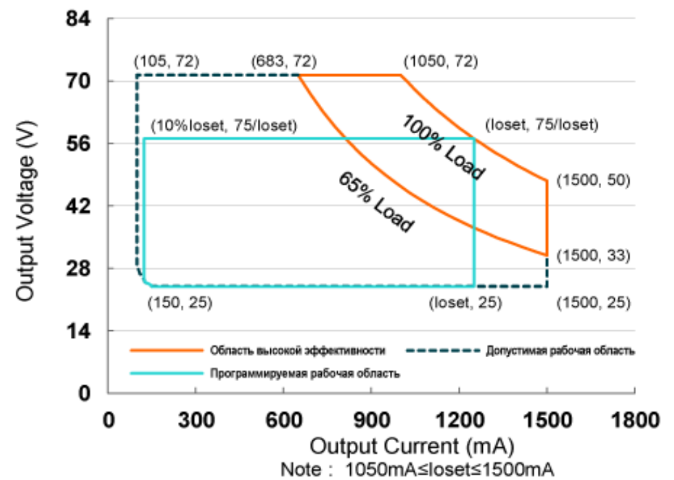
U/I график с областью Постоянная мощность
