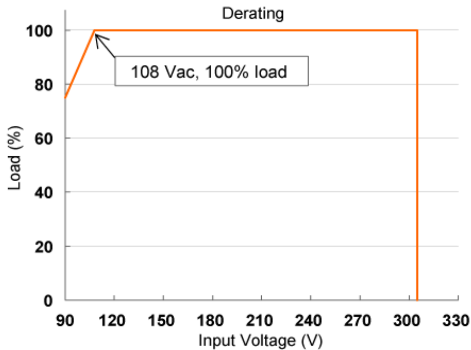
Зависимость вых. мощности от вх. напряжения
