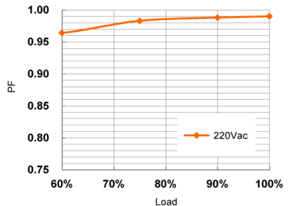
Коэффициент мощности
