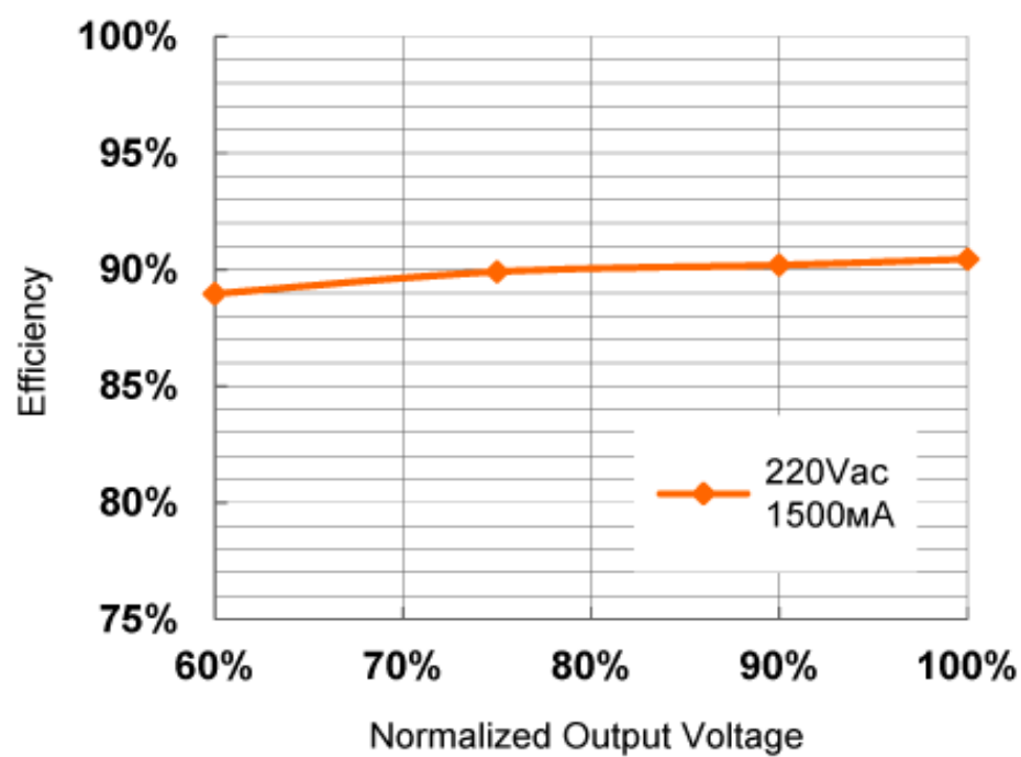
КПД в зависимости от нагрузки
