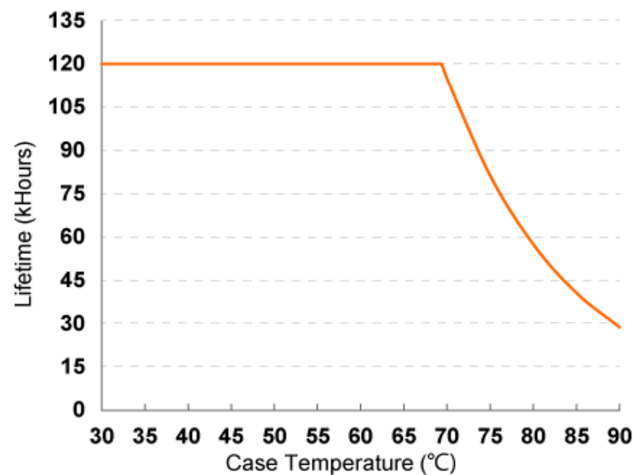
Срок службы / Температура на БП (T c )
