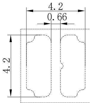
Fig.1-3 Bottom view 背面视图
